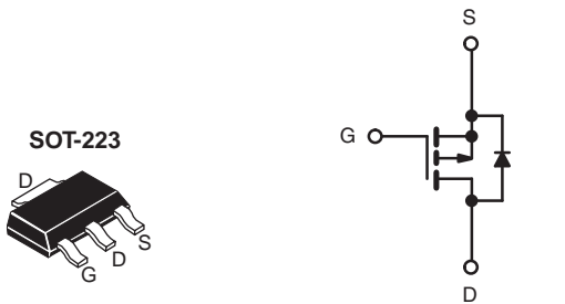
P-Channel MOSFET
