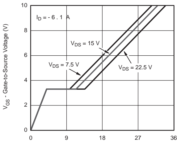
I_D = 6.1\text{ A} V_{DS} = 15\text{ V} V_{DS} = 7.5\text{ V} V_{DS} = 22.5\text{ V} Gate Charge
